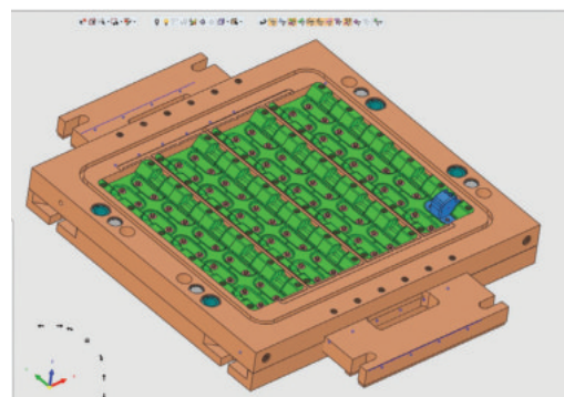
Spodná časť 40násobnej formy na doraz. Obstrek plechového dielca technickou gumou.
