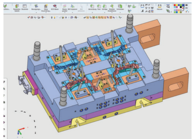
Pevná časť štvornasobnej formy s horúcim vtokom
